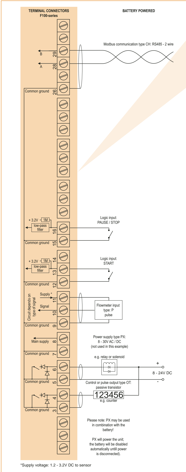
Typical wiring diagram F130-P-CH-PB-(PX)-OT
